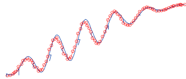
Mode 6V: f_e=2.26\text{Hz} , f_a=2.25\text{Hz}
