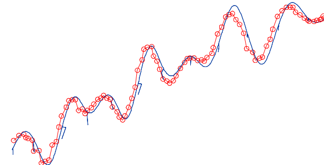
Mode 7V: f_e=2.43\text{Hz} , f_a=2.45\text{Hz}
